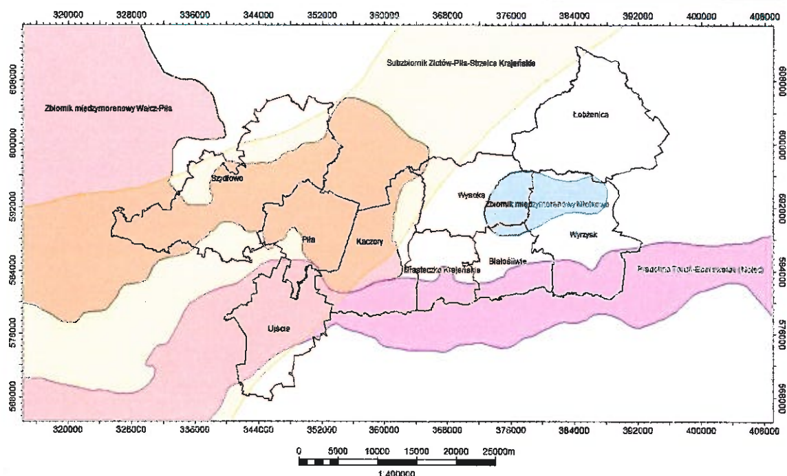
Rys. 3. Główne Zbiorniki Wód Podziemnych – fragment obejmujący Powiat Piliński
