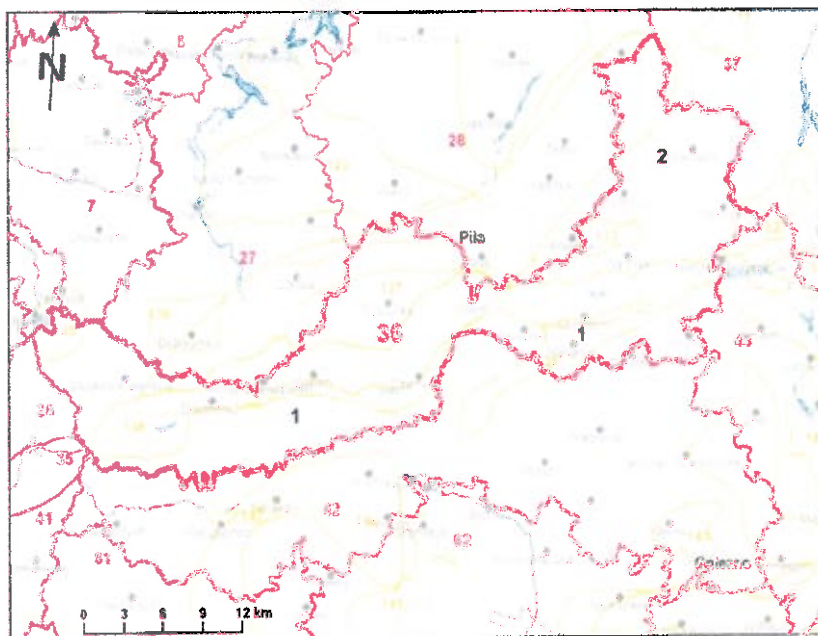
Rys.5. Jednolite Części Wód Podziemnych (JCWPd) - fragment mapy obejmujący Powiat Piliński
