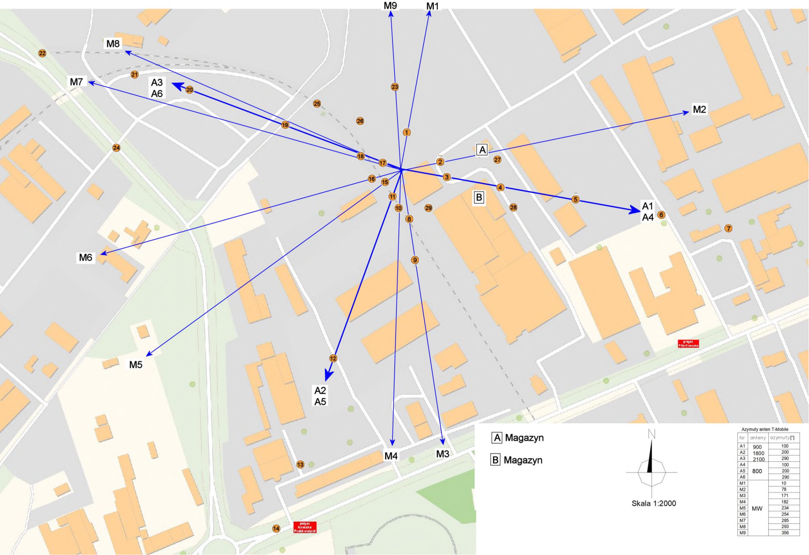
Zał. nr 2: Lokalizacja anten oraz ich azymuty, lokalizacja pionów (punktów) pomiarowych wokół instalacji radiokomunikacyjnej. -punkt (pion) ● pomiarowy.
